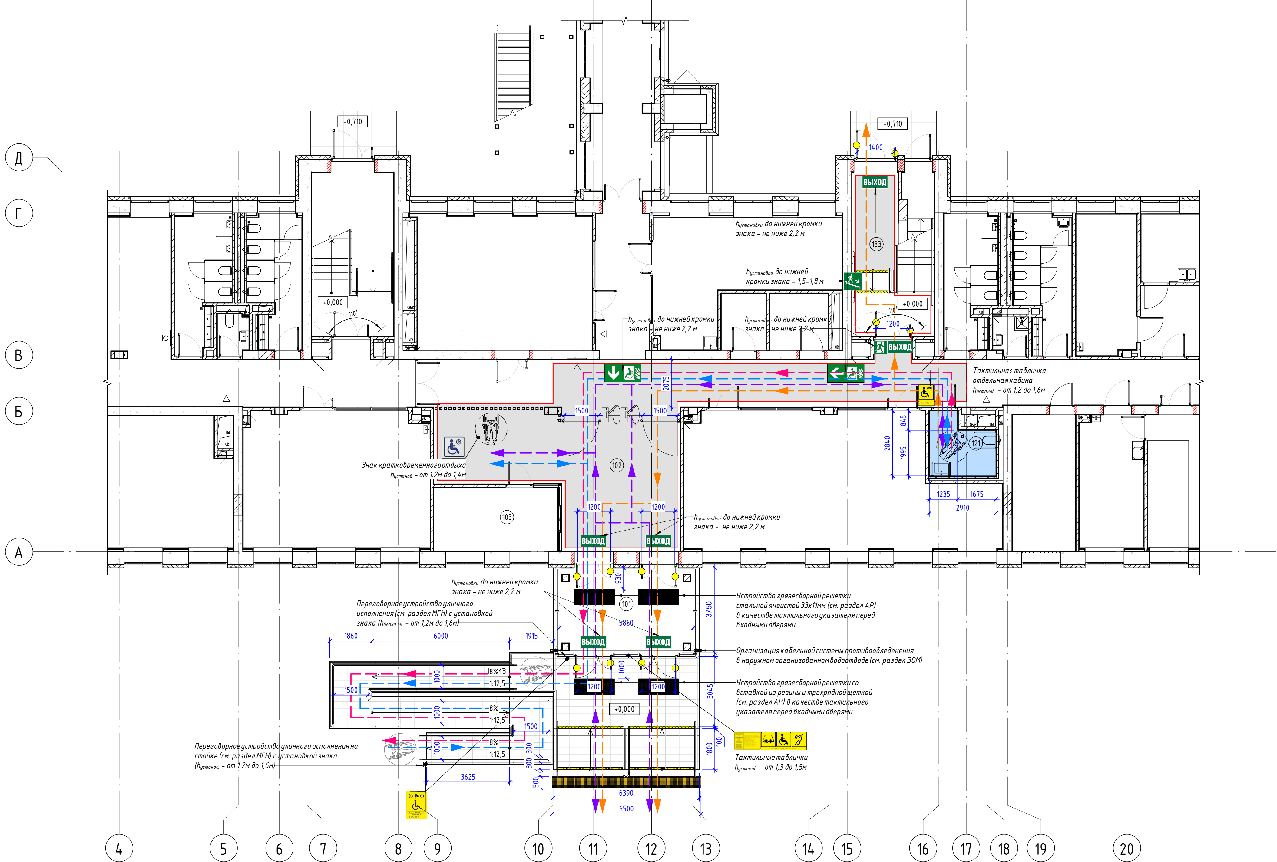
Фрагмент плана 1 этажа со схемой движения МГН
